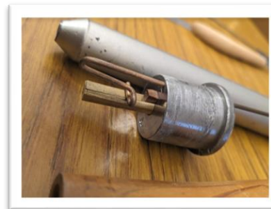
修復前のリードの状態
